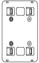
(150*117*15mm) 挂墙架
