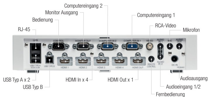
MS-1WL Multifunktions-Switcher/Scaler
